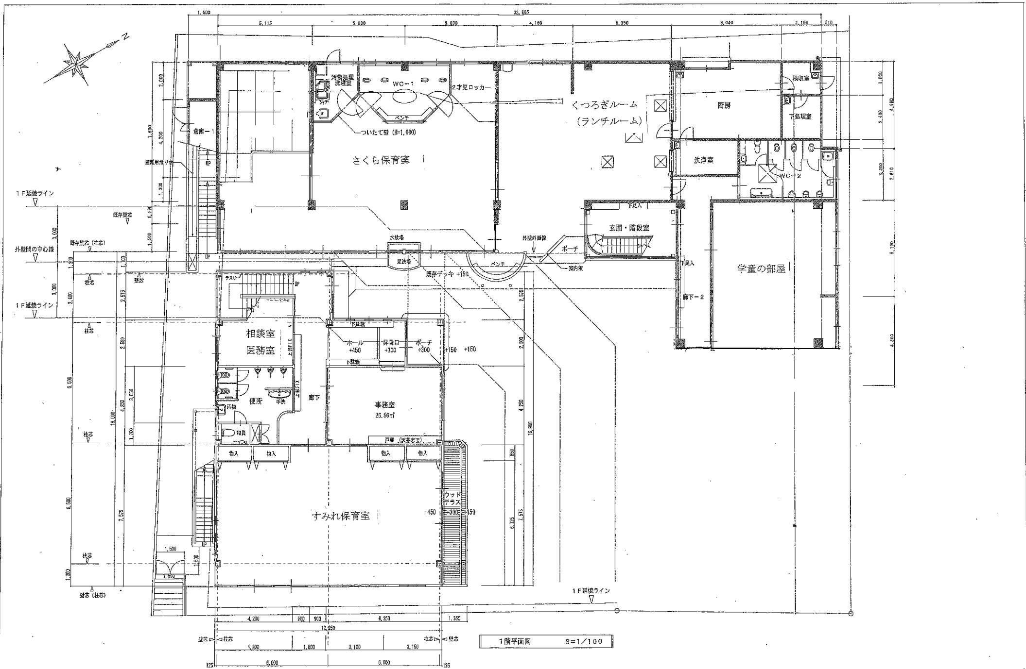
1階平面図
